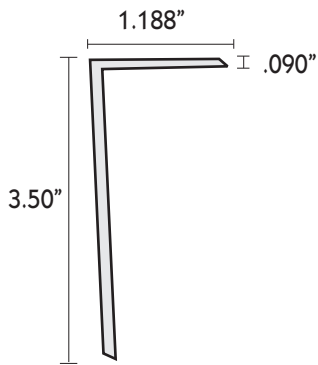
L-MOLDING
